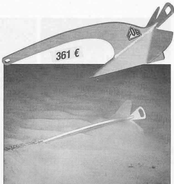
La géométrie très aboutie de la Rock se traduit par de bons résultats. Sur la courbe, on remarque notamment qu'elle ne commence à labourer que vers une tonne de traction.
