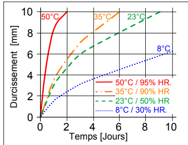
Diag1 : Vitesse de polymérisation des monocomposants Sikasil®
