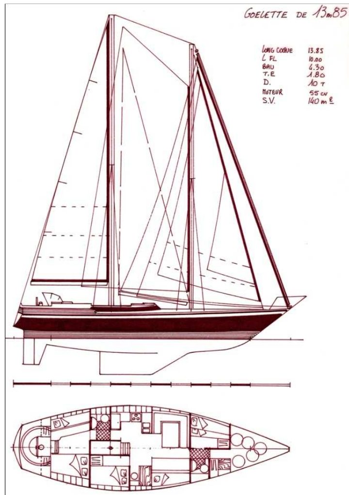
45' Polyester 14 x 4,30 m 1974
