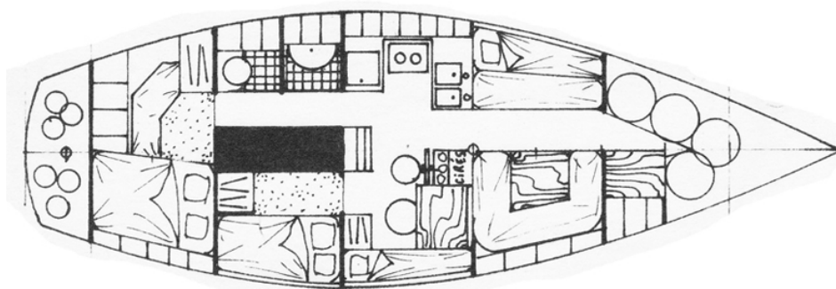
Aménagements de Mangareva (11,50 / 12 x 4,14 m 1973) Ce sont aussi les dispositions proposées pour le 37/40
