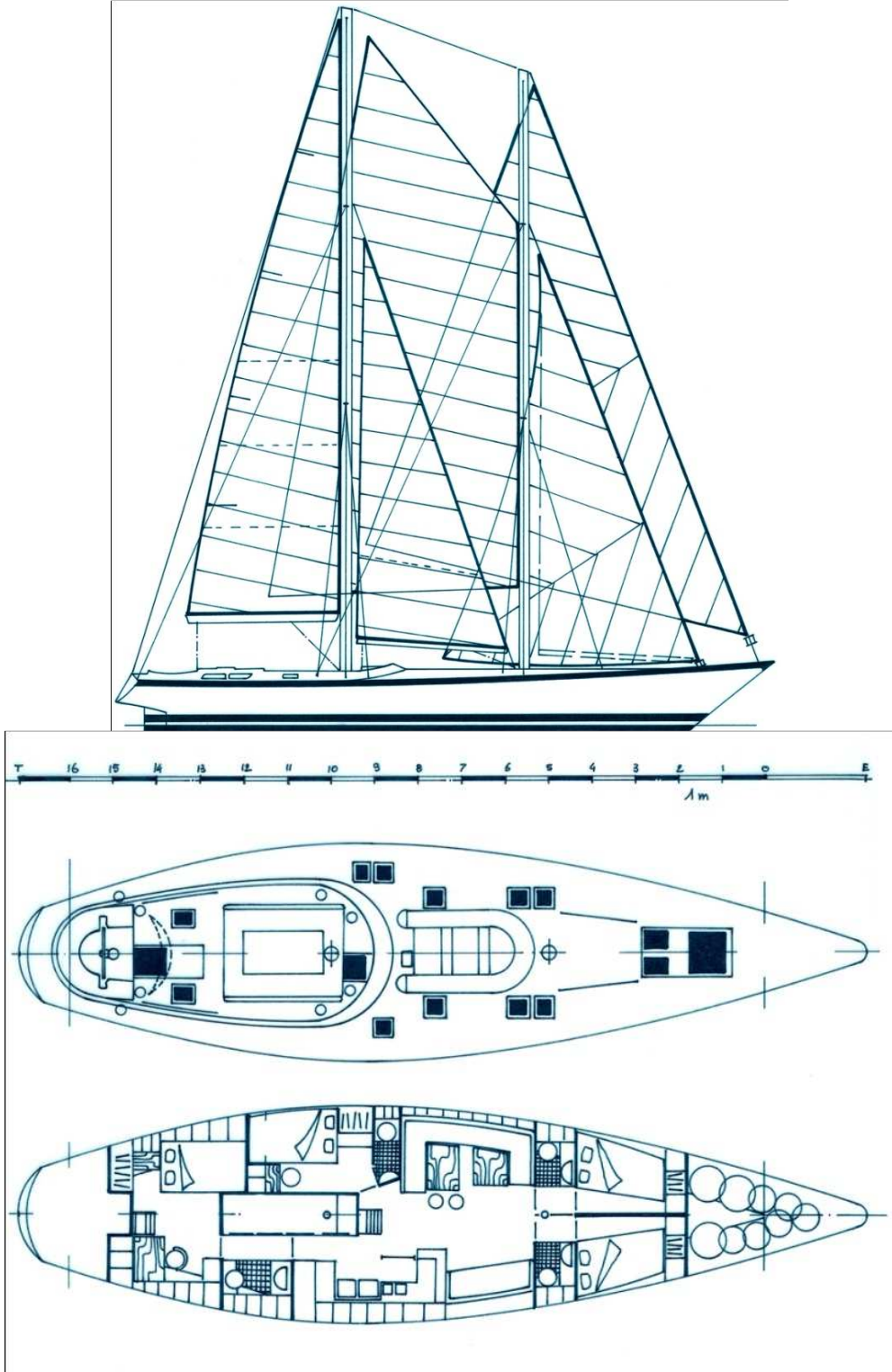
Kreis An Ael 20 m x 5 m 1977
