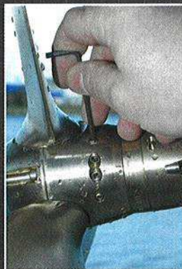
▲ On règle le pas (avant/arrière) avec une clé à lène.
