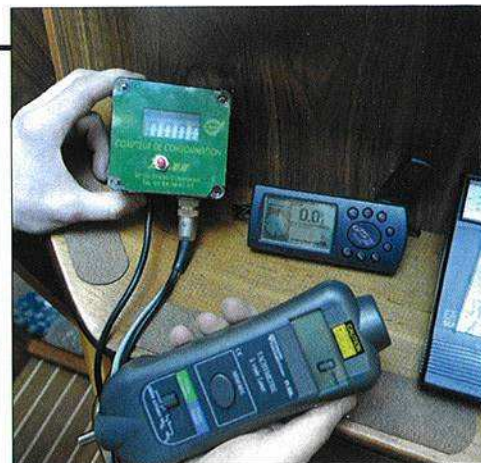
▲ Tachymètre à visée laser, débitmètre digital, sonomètre et GPS : rien n'a été laissé au hasard.
