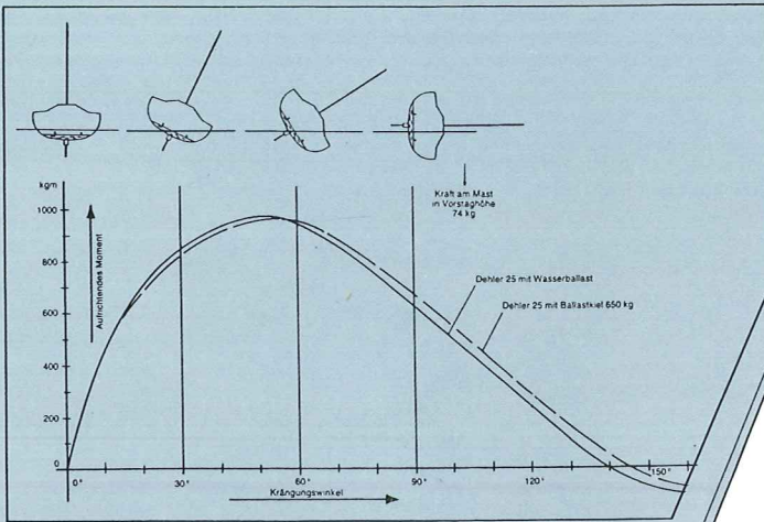
Die in der YACHT Nr. 1/83 gezeigte Grafik mit Vergleichszahlen zwischen dem Wasserballast-System und einem normalen Festkiel zeigt, daß die Stabilitätswerte beim Wasserballast-System gleich gut sind.
