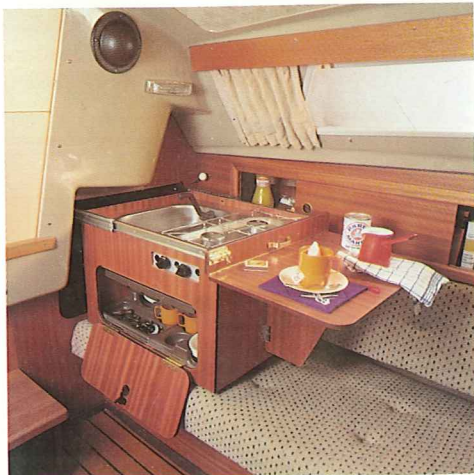
Diese fahrtgerechte Pantry**) hat einen zwei-flammigen Gasherd*), Spüle und einen geräumigen Geschirrschrank. Nach Gebrauch wird sie unter die Backbord-Sitzducht geschoben.
