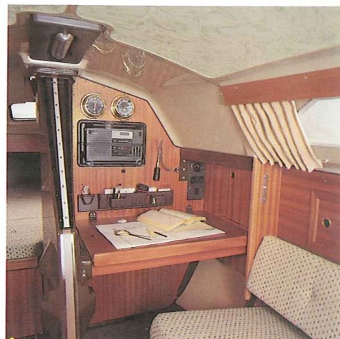
An Steuerbord liegt der separate Navigationsplatz mit Kartenfach und Schrank.
