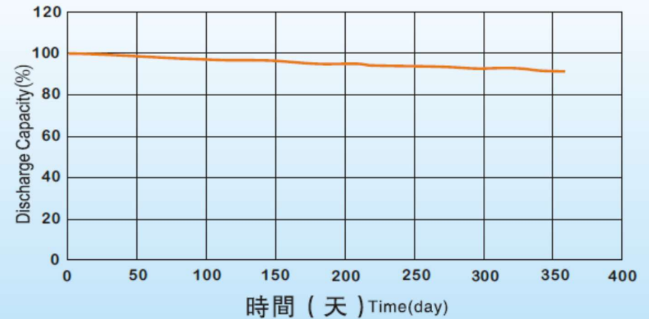
在常溫下LYP類電池的存儲特性曲綫
